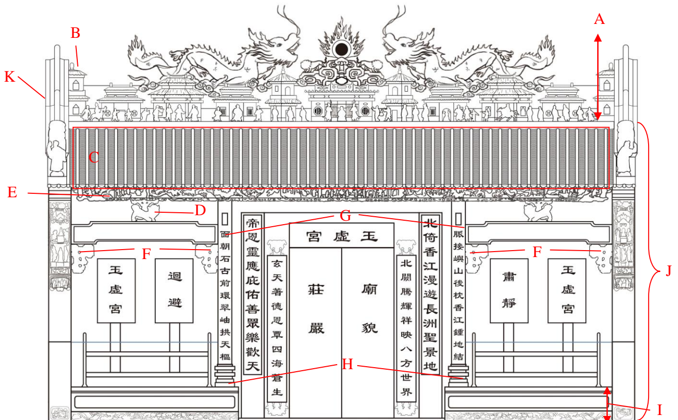
圖 3 立面圖
