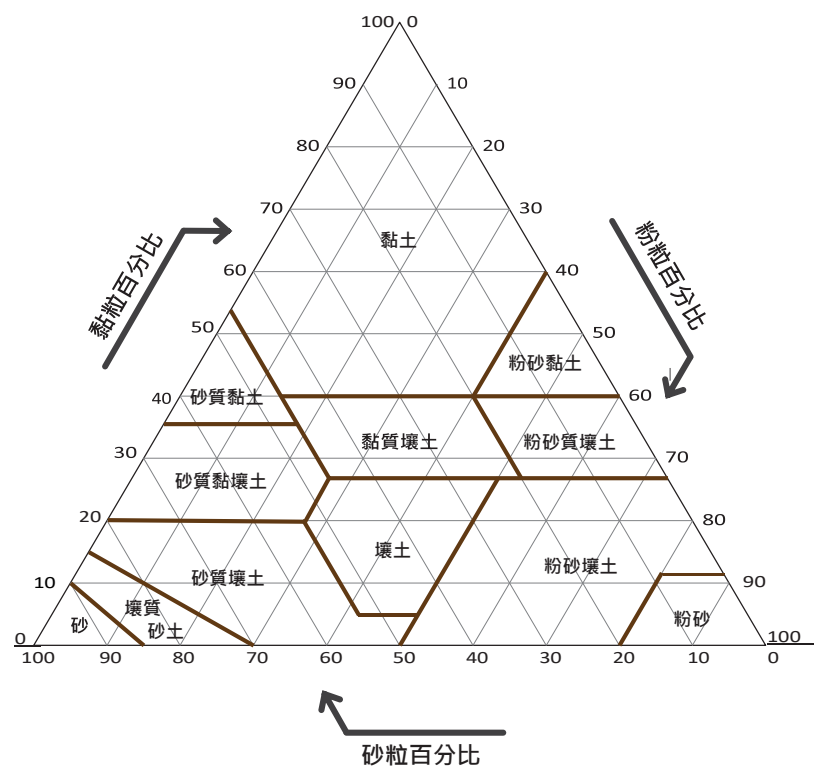
圖 2. 土壤質地三角表
