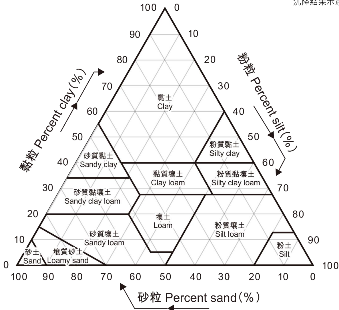
圖：土壤質地三角形圖
